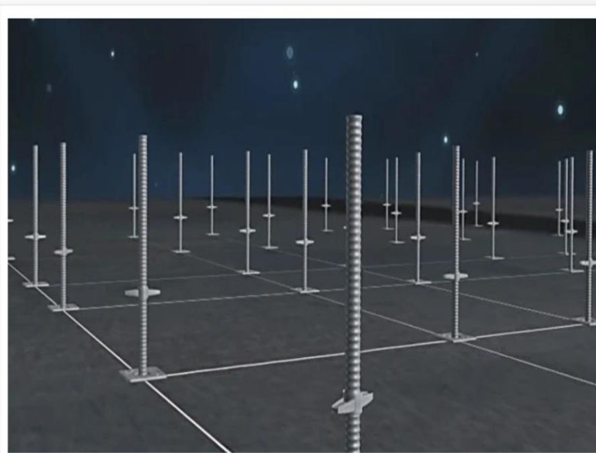
可调底座（立杆）安放
